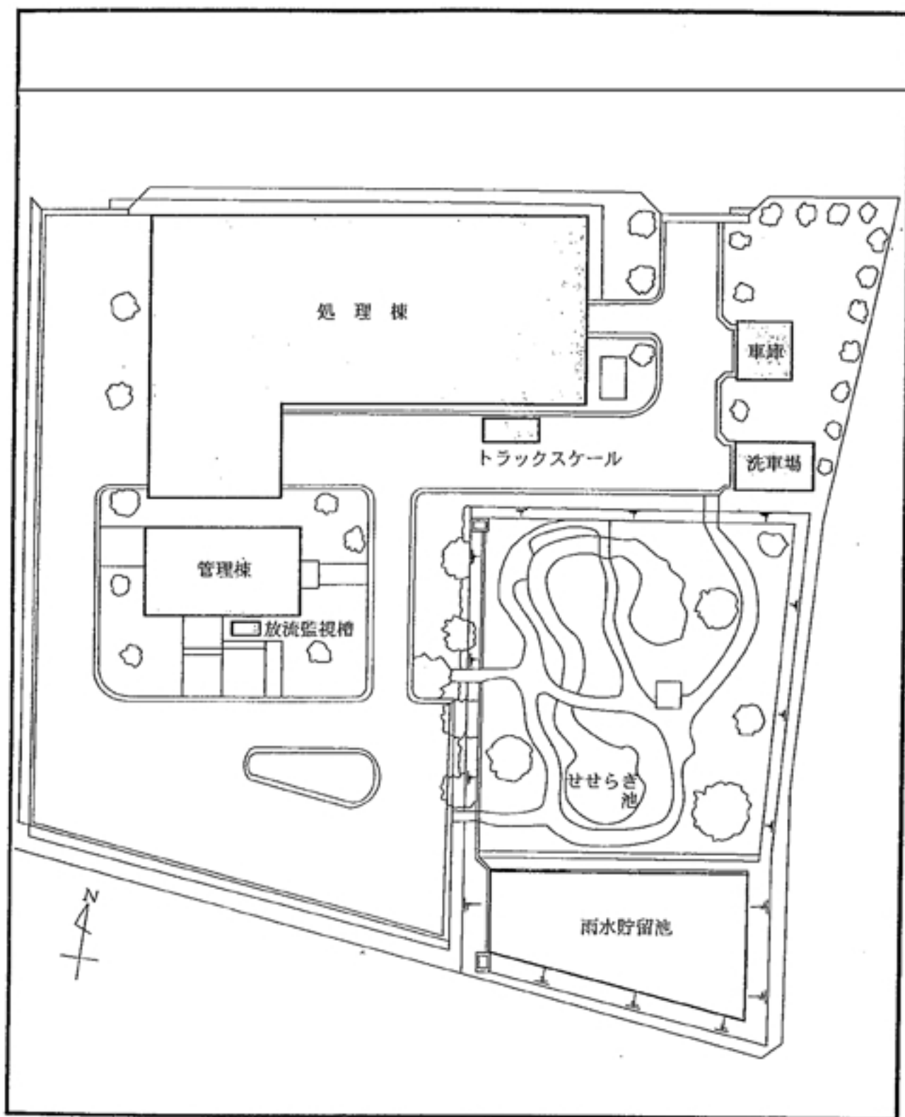
全体配置図
